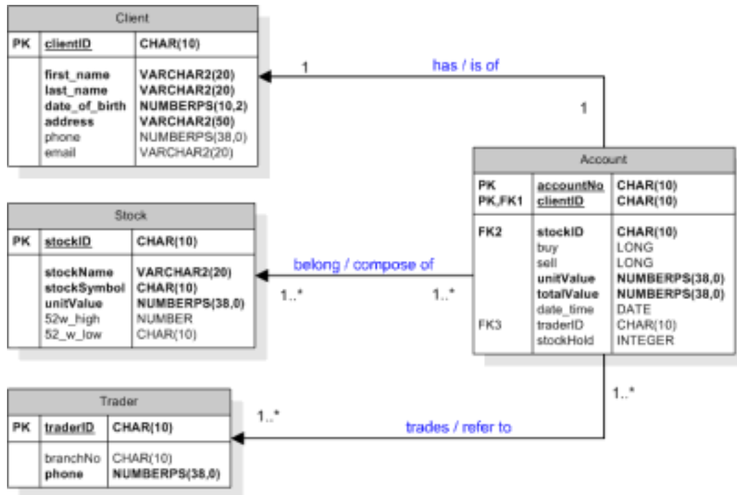
Revised ER model
